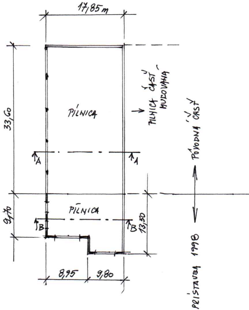
REZ A-A
